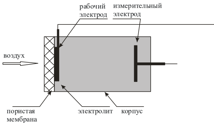
Рис. 1. Электрохимический детектор
